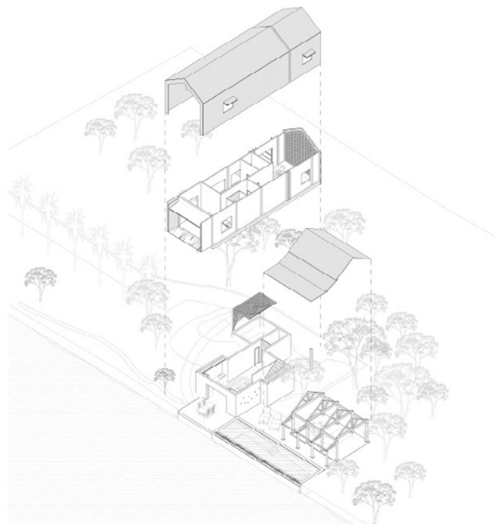
AXONOMETRIC
