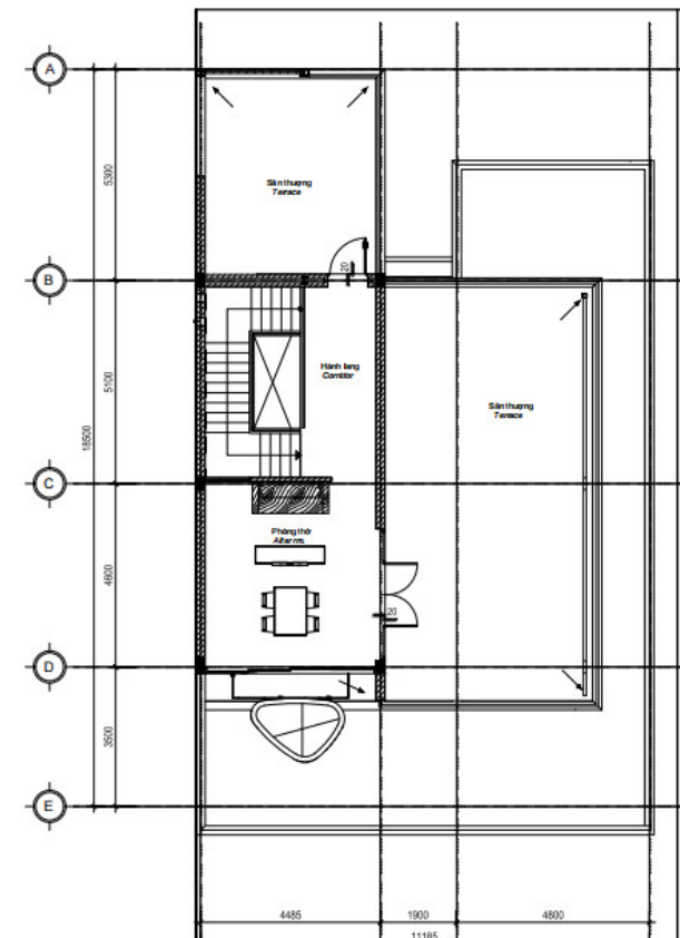
TẦNG 3
