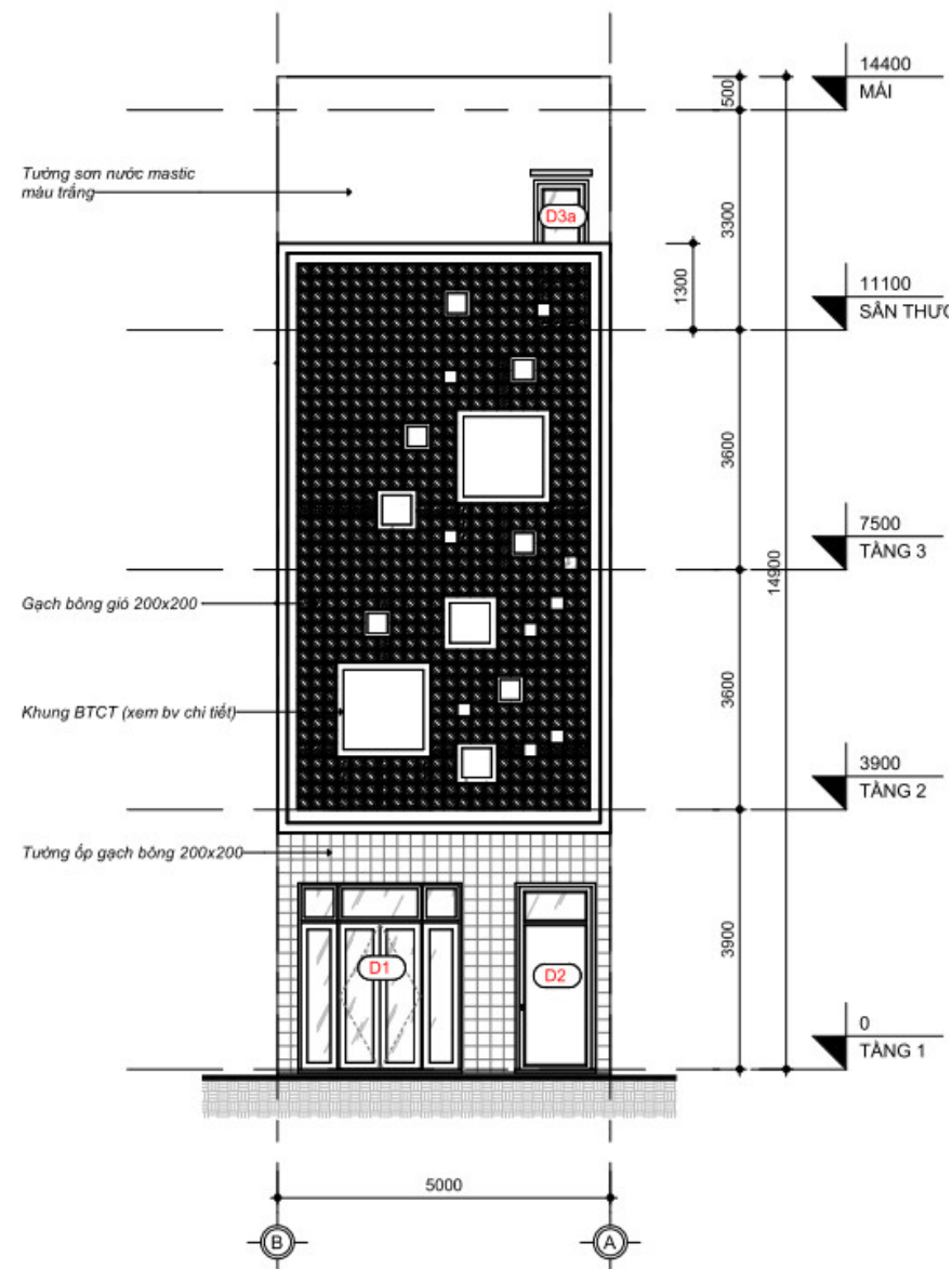
1 MẶT ĐỨNG TRỰC B - A/ B-A EXTERIOR ELEVATION 1:100
