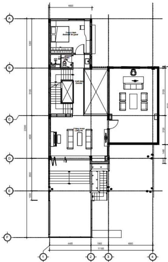
TẦNG 1
