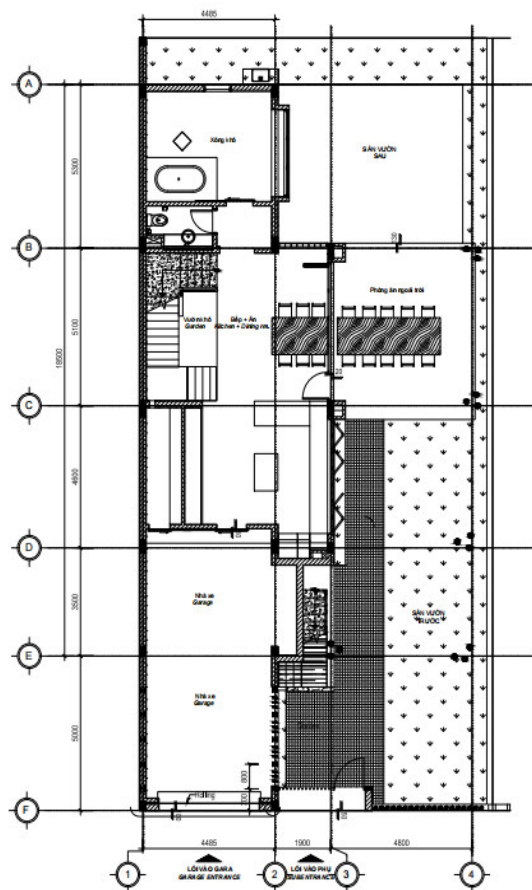
TẦNG TRỆT
