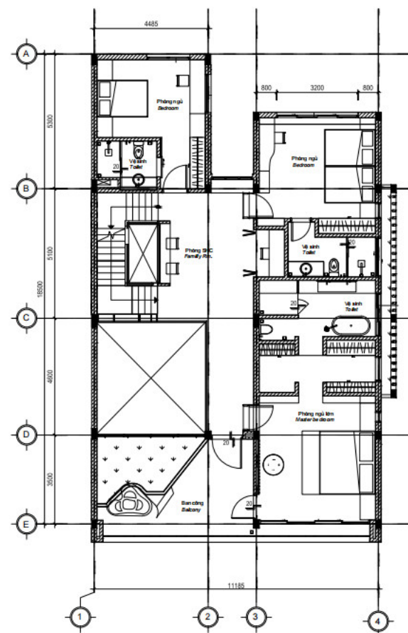
TẦNG 2
