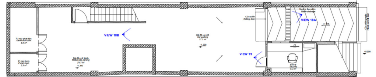
Basement | Tầng Hầm
